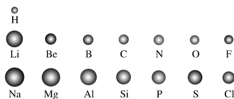
短周期主族元素原子半径的周期性变化
